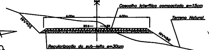
SEÇÃO TRANSVERSAL TIPO MISTA
