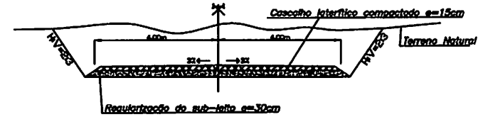
SEÇÃO TRANSVERSAL TIPO EM CORTE
