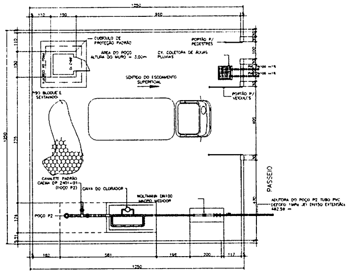
PLANTA DE URBANIZAÇÃO POÇO 02.03.04
