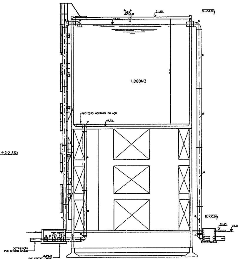
CORTE AB
