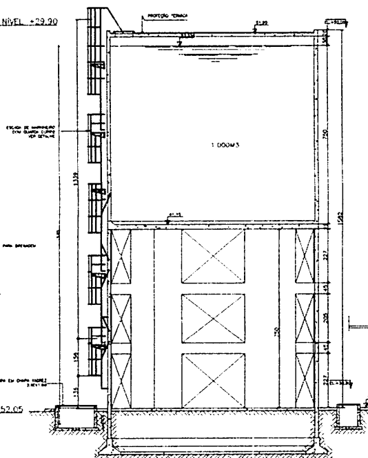
CORTE AB ESCALA 1/25
