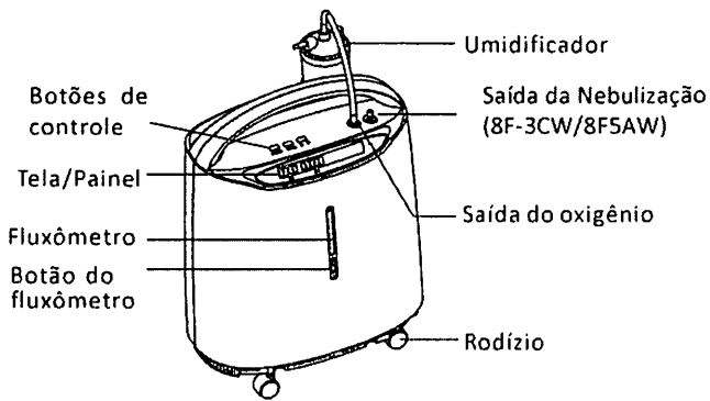
Figura 1: Visão completa (frente)
