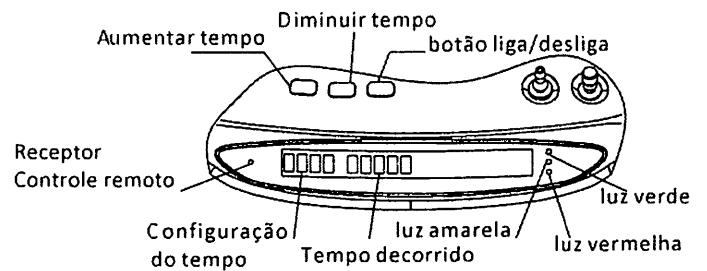
Figura 3: painel de controle
