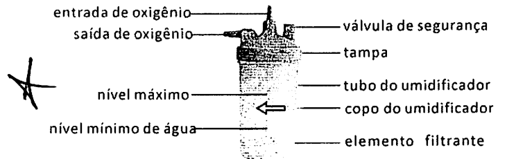
Figura 4: componentes do umidificador
