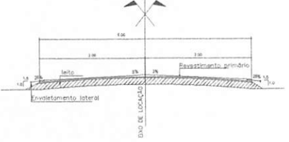
SEÇÃO TIPO - TRANSVERSAL
