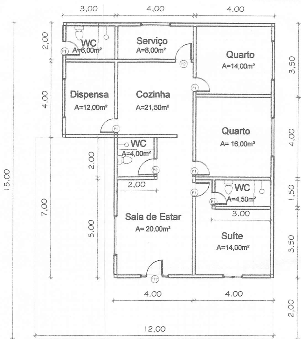
1 Planta Baixa 1 : 100
