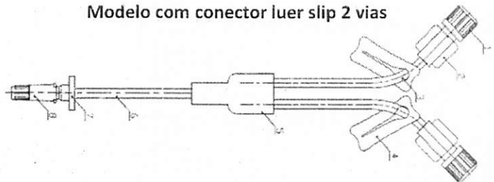
Modelo com conector luer slip/lock 2 vias
