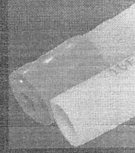
Sonda de Foley
